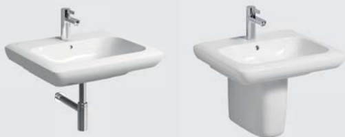
Waschtisch, 600 x 480 mm, Modell-Nr. 121960. Kombinierbar mit Halbsäule, Modell-Nr. 291910 oder Waschtischunterschränken 494 mm.
