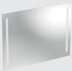
Lichtspiegelement , mit integriertem Lichtschalter, T5, 2 x 24 W, 4000 K, 230 V, ~50 Hz, IP44, Schutzklasse 2, Energieklasse A, 900 x 650 x 36 mm, Modell-Nr. 800490.
