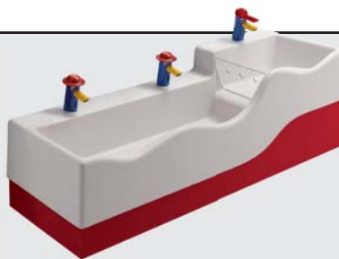
3Bambini Spiel- und Waschlandschaft, Version links, mit 3 Waschplätzen, aus Varicor®, mit herausnehmbarer Wasserstauscheibe, 1390 x 300 x 415 mm, Modell-Nr. 430300016 Weiß (Alpin). Kombinierbar mit Front- und Seiten-Dekorblenden aus Varicor® in den Farben Blau, Rot, Gelb, Grün, Weiß und Orange sowie mit 4Bambini Infrarotarmatur oder Einhebelmischer.
