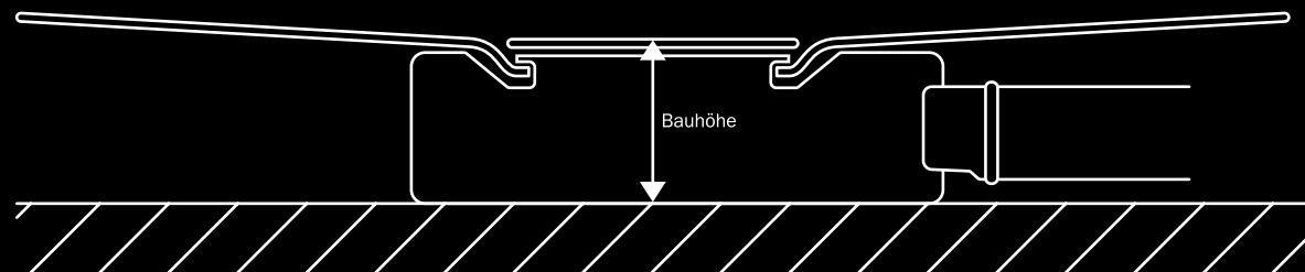
Schematische Darstellung der SCONA mit KA 90
