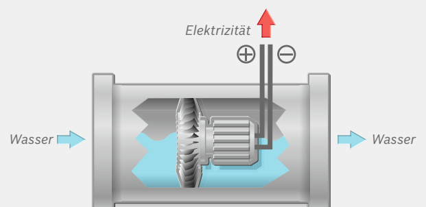
Funktionsprinzip Hydro-Power-Technologie
