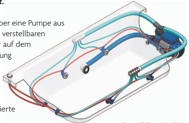
Systemabbildung Hydro 5000
