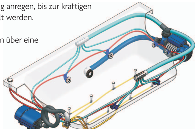
Systemabbildung Combi 5000
