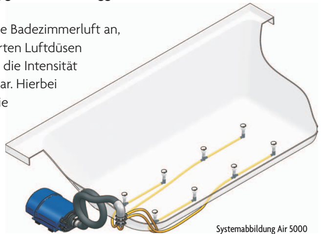
Systemabbildung Air 5000
