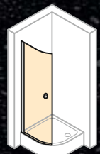
1/4 Kreis Schwingtür 2-flügelig
