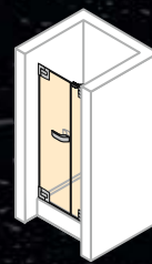
Schwingtür mit Nebenteil in Nische
