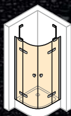
1/4 Kreis Schwingtür mit festen Segmenten 2-flügelig
