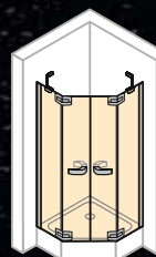
5-Eck Schwingtür mit festen Segmenten, 2-flügelig
