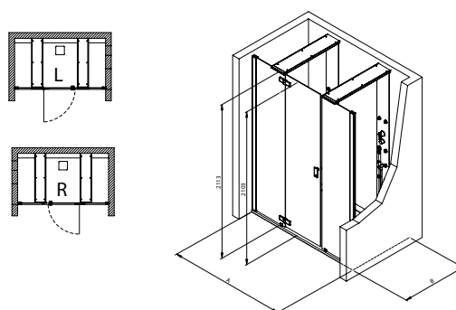
Thasos for two für Nische / Niche
