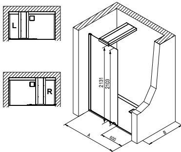
Ciela für Nische / Niche
