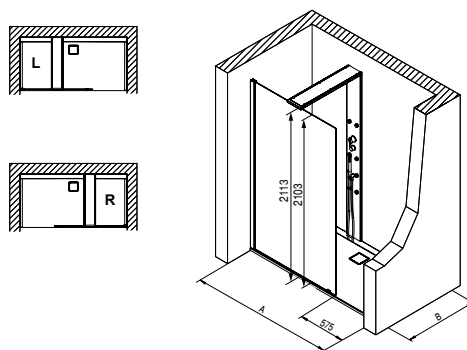
Thasos für Nische / Niche
