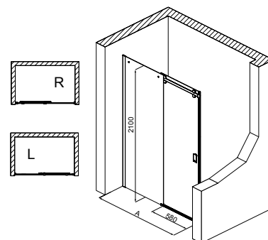
Muna für Nische / Niche
