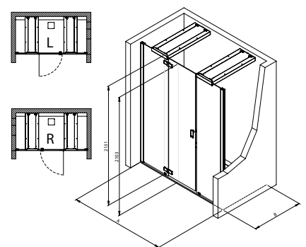
Ciela for two für Nische / Niche
