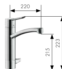
Einhebel-Küchenmischer mit Absperrventil Art.-Nr. 31783000
