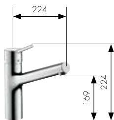
Einhebel-Küchenmischer Art.-Nr. 32851, -000, -800 für offene Warmwasserbereiter Art.-Nr. 32852000
