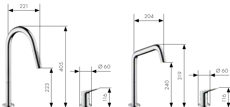
2-Loch Einhebel-Küchenmischer mit Ausziehbrause Art.-Nr. 34822, -000, -800
