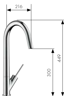
Einhebel-Küchenmischer mit Schwenkauslauf
