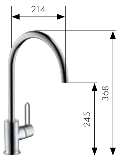
Einhebel-Küchenmischer mit Schwenkauslauf Art.-Nr. 38830, -000, -800
