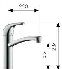
Einhebel-Küchenmischer Art.-Nr. 31780000 für offene Warmwasserbereiter Art.-Nr. 31784000
