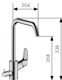
Einhebel-Küchenmischer mit Schwenkauslauf und Absperrventil Art.-Nr. 31823000
