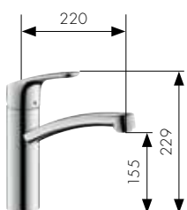
Einhebel-Küchenmischer Art.-Nr. 31806, -000, -800 für offene Warmwasserbereiter Art.-Nr. 31804000
