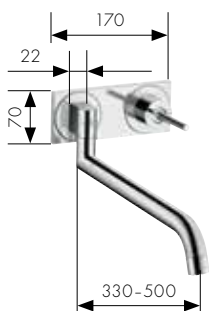
Einhebel-Küchenmischer, Unterputz Art.-Nr. 38815, -000, -800 Grundkörper (o. Abb.) Art.-Nr. 13622180
