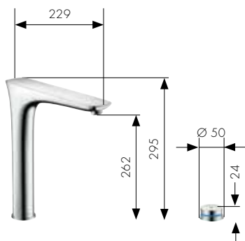
2-Loch Elektronik-Küchenmischer Art.-Nr. 15805, -000, -800
