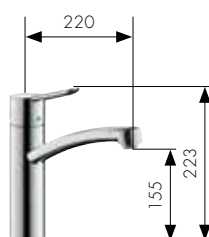
Einhebel-Küchenmischer Art.-Nr. 31786000 für offene Warmwasserbereiter Art.-Nr. 31785000
