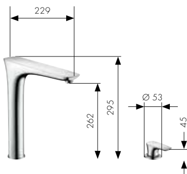
2-Loch Einhebel-Küchenmischer Art.-Nr. 15812, -000, -800
