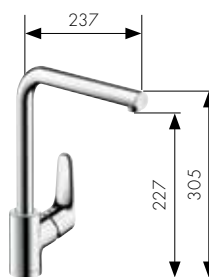
Einhebel-Küchenmischer mit Schwenkauslauf (L-Auslauf) Art.-Nr. 31817, -000, -800
