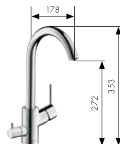
Einhebel-Küchenmischer mit Schwenkauslauf und Absperrventil Art.-Nr. 14875000
