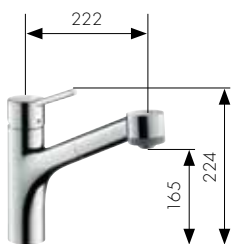
Einhebel-Küchenmischer mit Ausziehbrause Art.-Nr. 32841, -000, -800 für offene Warmwasserbereiter Art.-Nr. 32842000
