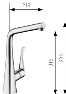
Einhebel-Küchenmischer mit Schwenkauslauf Art.-Nr. 14822, -000, -800 für Montage vor Fenstern Art.-Nr. 14823000
