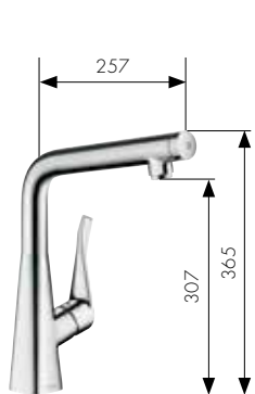
Einhebel-Küchenmischer mit Schwenkauslauf Art.-Nr. 14883, -000, -800
