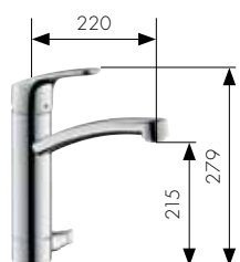
Einhebel-Küchenmischer mit Absperrventil Art.-Nr. 31803000
