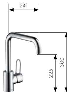
Einhebel-Küchenmischer mit Schwenkauslauf Art.-Nr. 14850000 für offene Warmwasserbereiter Art.-Nr. 14852000 mit Absperrventil (o. Abb.) Art.-Nr. 14855000
