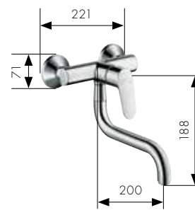
Einhebel-Küchenmischer für Wandmontage Art.-Nr. 31825000
