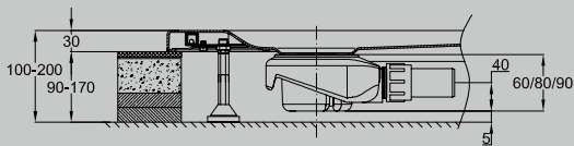
Abb.: mit seitlicher Entwässerung
