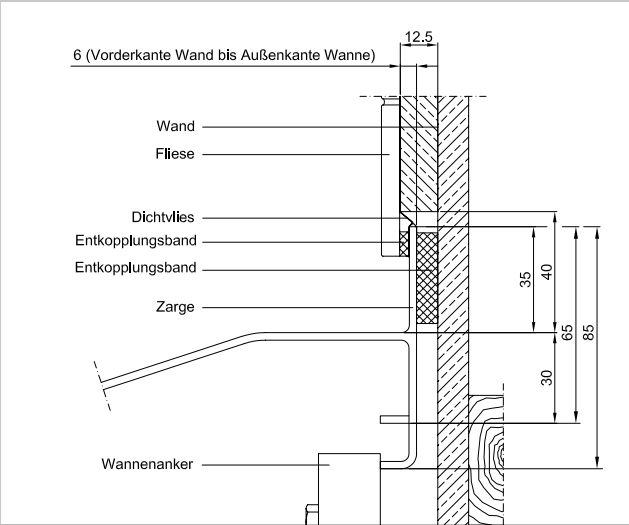
Darstellung Leichtbauwand
