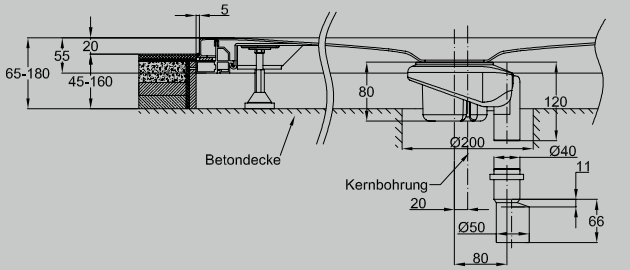
Abb.: mit senkrechter Entwässerung
