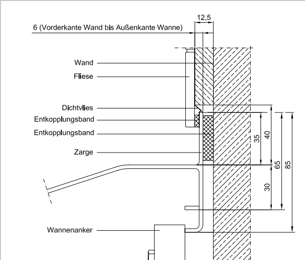
Darstellung Massivbauwand
