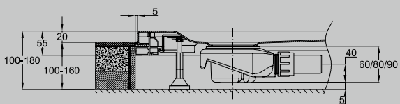
Abb.: mit seitlicher Entwässerung
