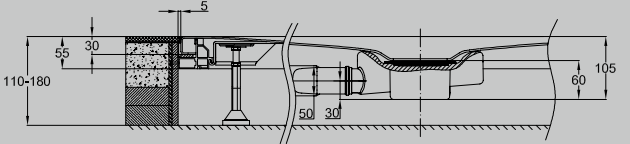
Abb.: mit seitlicher Entwässerung
