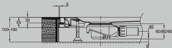
Abb.: mit seitlicher Entwässerung
