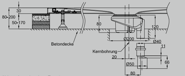
Abb.: mit senkrechter Entwässerung
