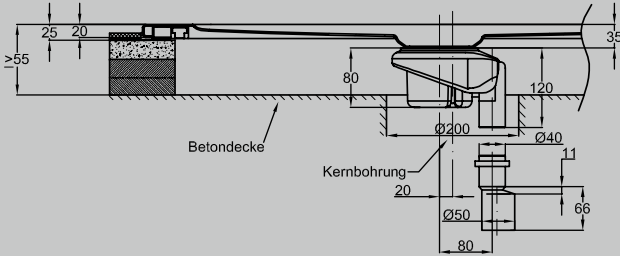
Abb.: mit senkrechter Entwässerung
