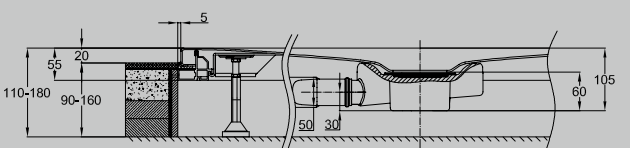
Abb.: mit seitlicher Entwässerung
