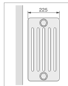
6-Säuler (Bautiefe - 225 mm)
