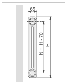
2-Säuler (Bautiefe - 65 mm)
