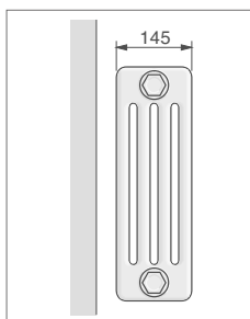
4-Säuler (Bautiefe - 145 mm)
